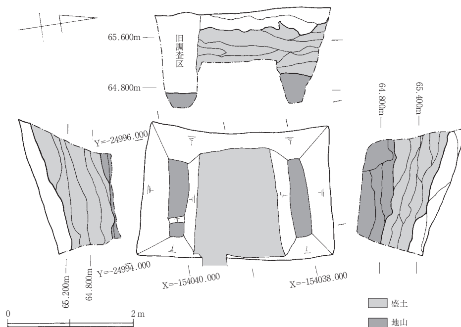
図6 第5調査区平面図・断面図 1:30
