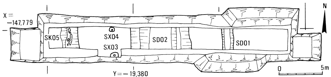
第34図 薬師寺旧境内(1)発掘遺構図
