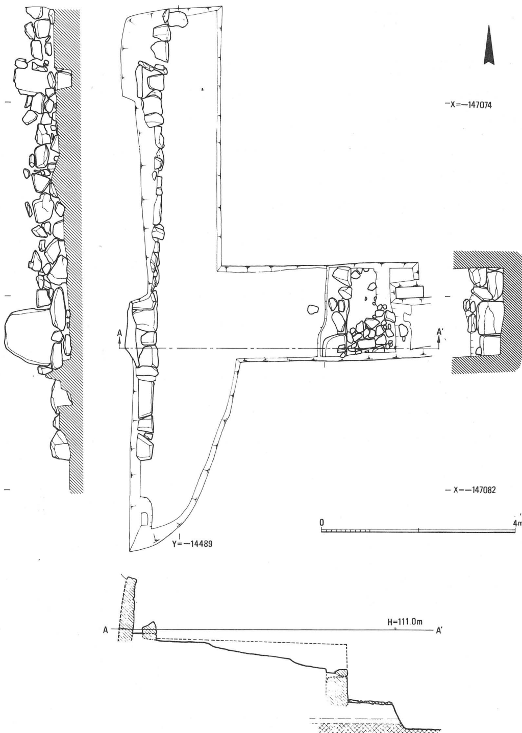
第13図 頭塔調査遺構平面・立面・断面図
