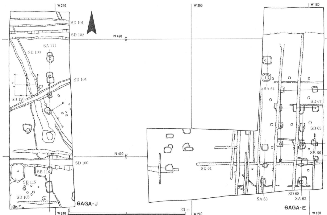
第12図 第 103 - 7 次調査遺構図
