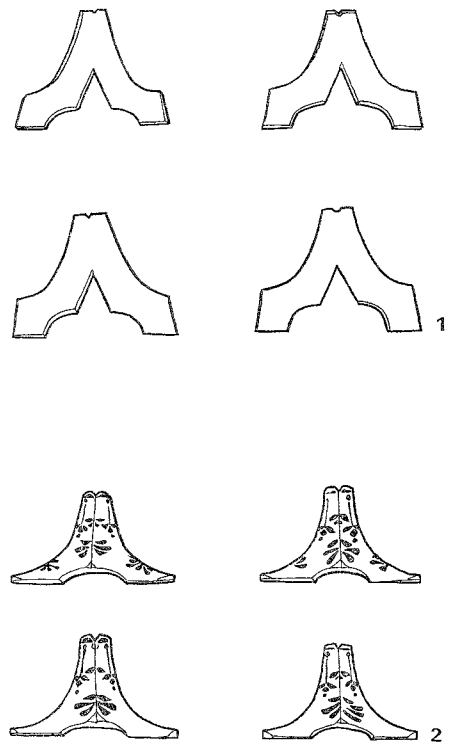
fig. 45 正倉院の琴柱 1; 金泥絵新羅琴 2; 金箔押新羅琴 (前掲『正倉院の木工』図版147・148)
