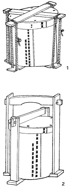
fig. 41 把手と枠の復原
