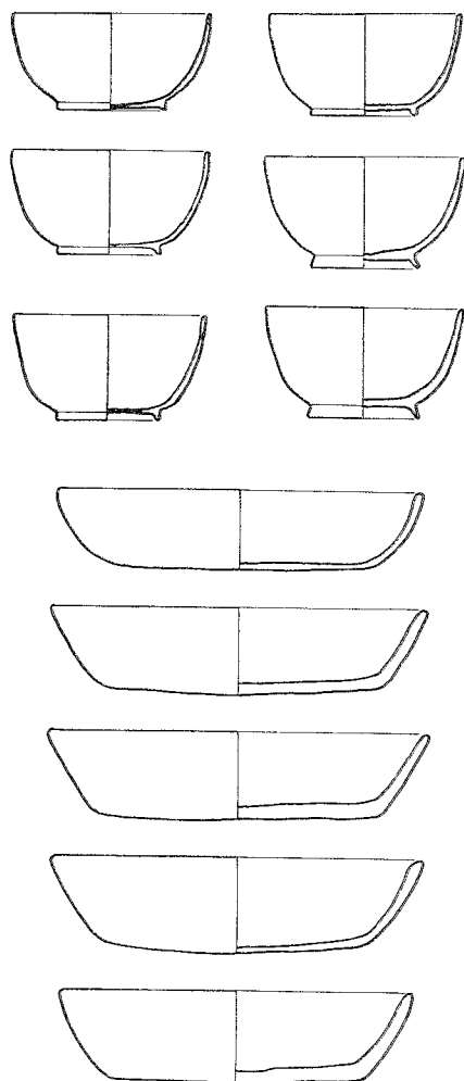
fig. 28 正倉院の漆食器 (前掲『正倉院の漆工』実測図3・6 1:4)
