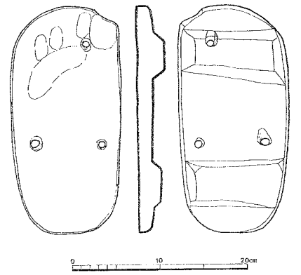
fig. 26 A II a 型式の下駄 兵庫県山垣遺跡東堀出土 8 世紀前葉
