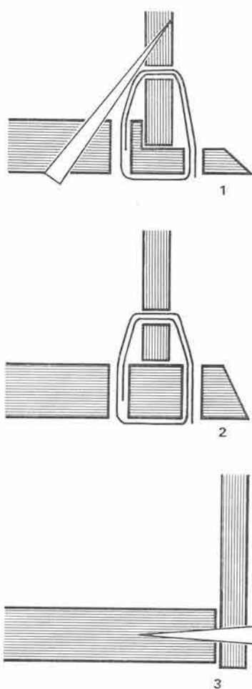
fig. 33 曲物の結合模式図
