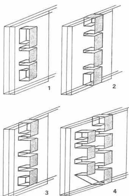
fig. 32 曲物の綴方模式図
