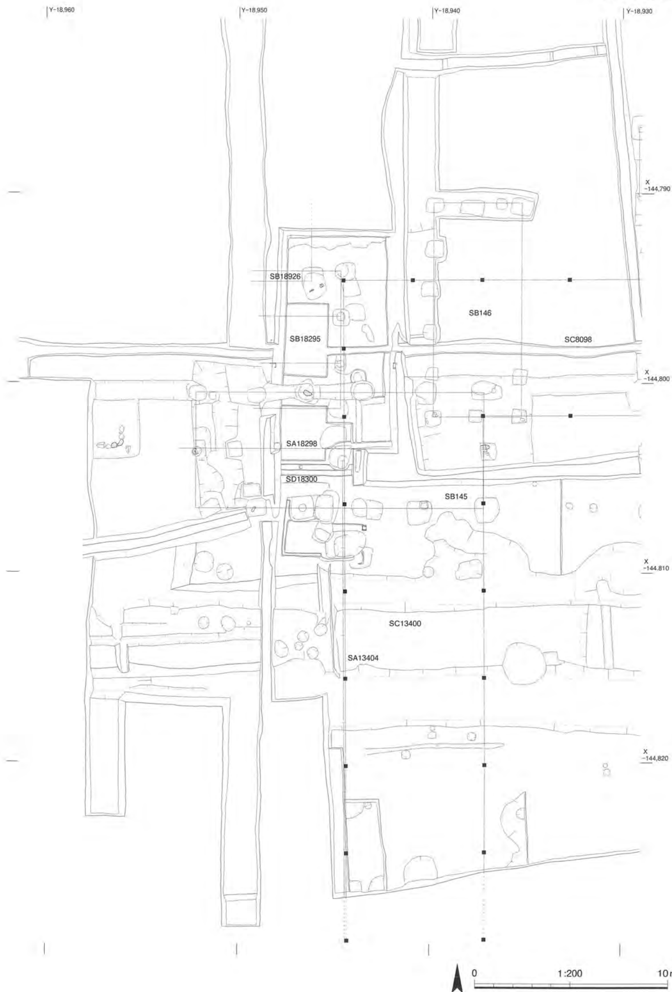
遺構実測図2
