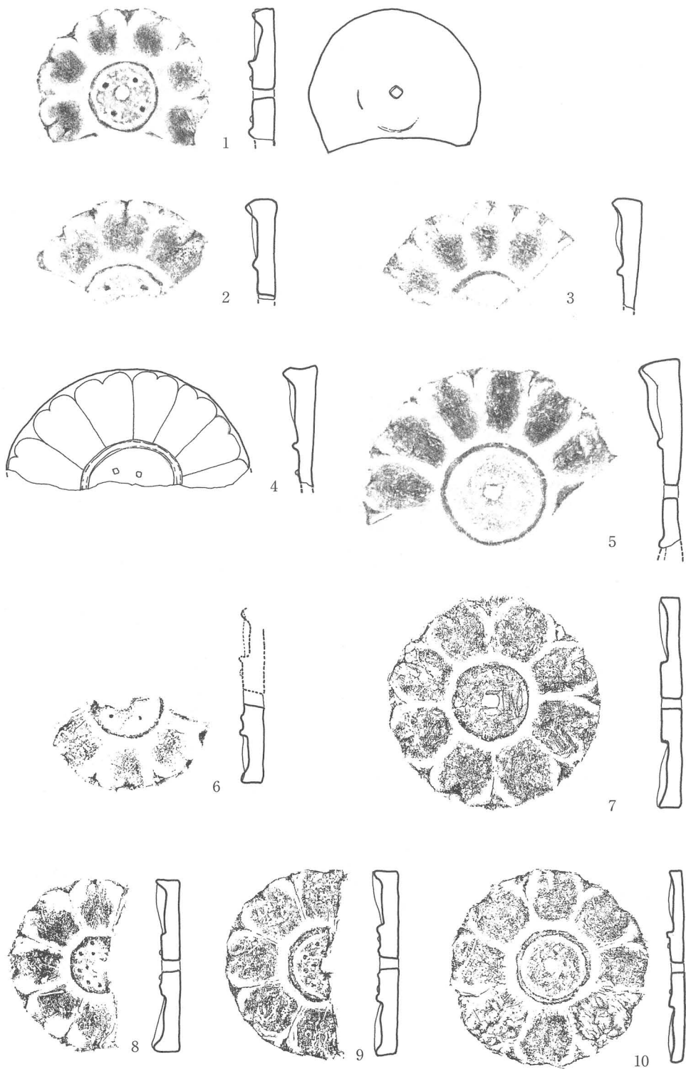
第1図 百済の垂木先瓦 (1:4) 1~5: 定林寺址、6: 亭岩里窯、7~10: 陵山里寺址
