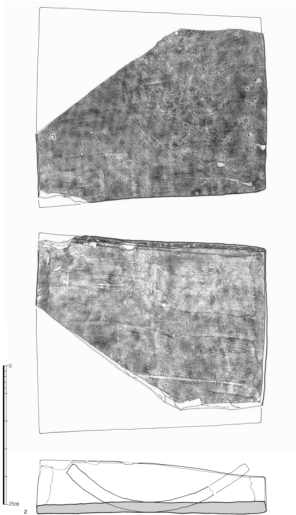
Fig. 73 平瓦1類実測図(2) 1:4
