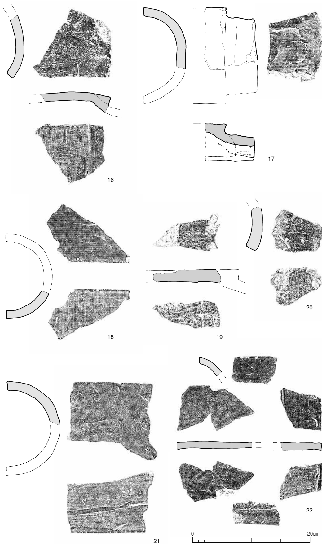
Fig. 71 丸瓦実測図 (5) 1:4
