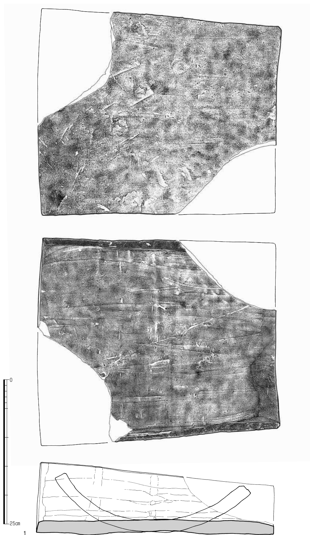
Fig. 72 平瓦1類実測図(1) 1:4
