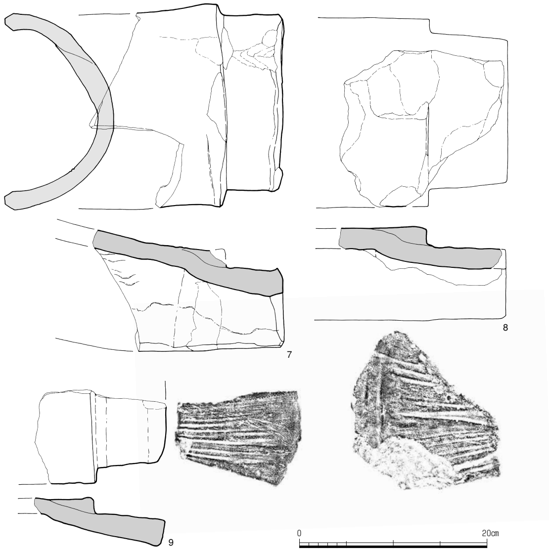
Fig. 69 丸瓦実測図 (3) 1:4
