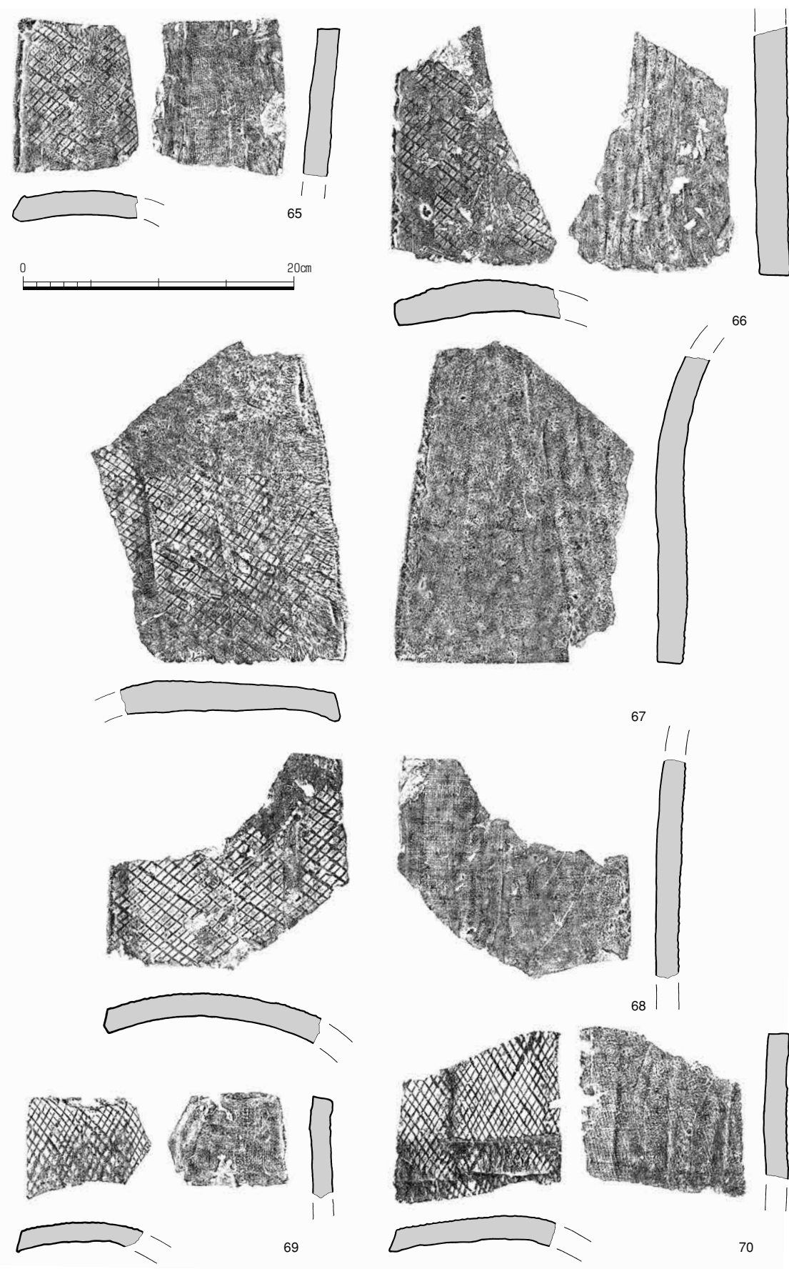
Fig. 86 平瓦5類拓影 1:4
