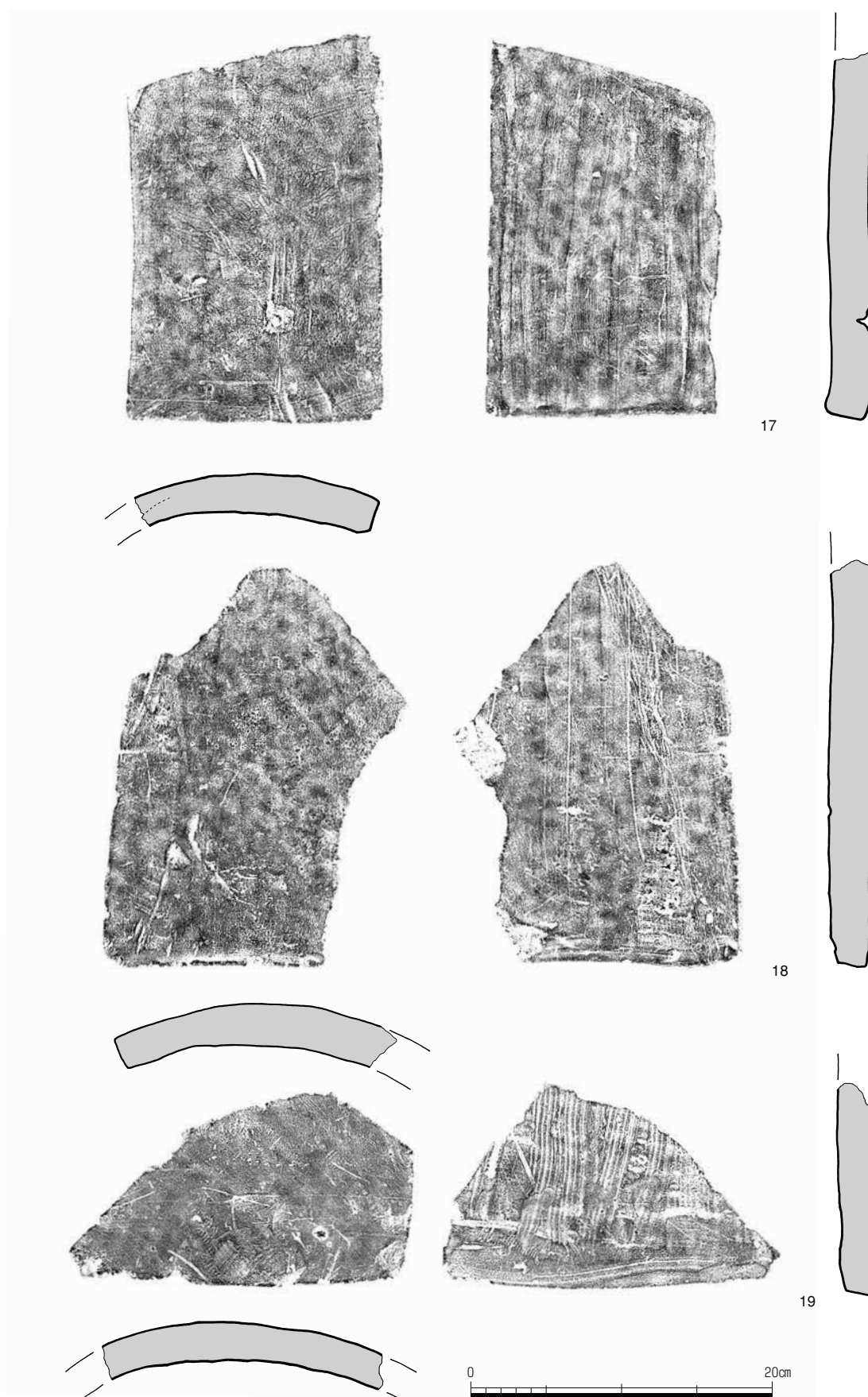
Fig. 79 平瓦1類拓影(5) 1:4
