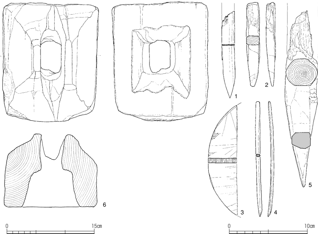
Fig. 101 木製品 1:3 (6のみ1:4)
