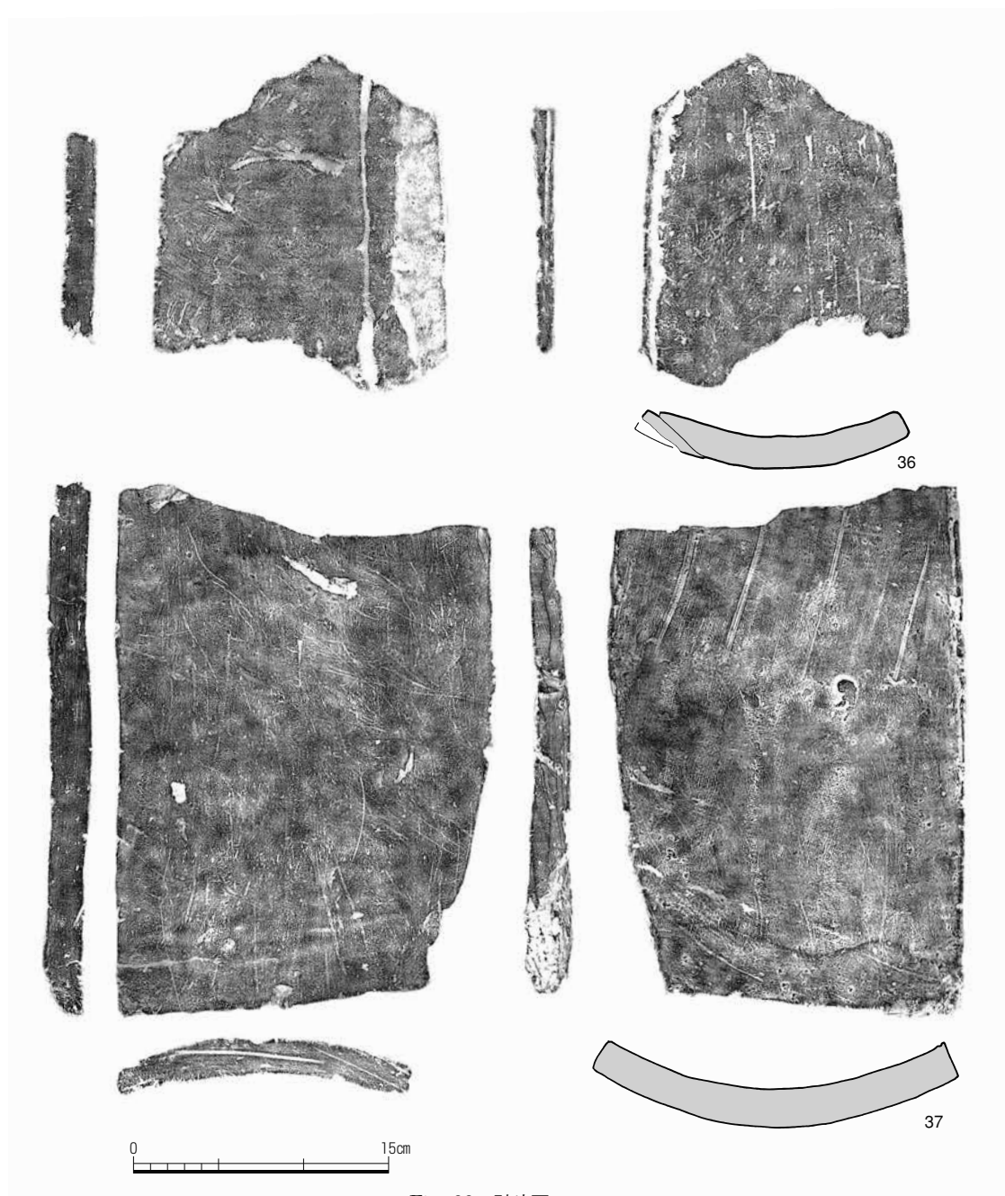
Fig. 66 熨斗瓦 1:4
