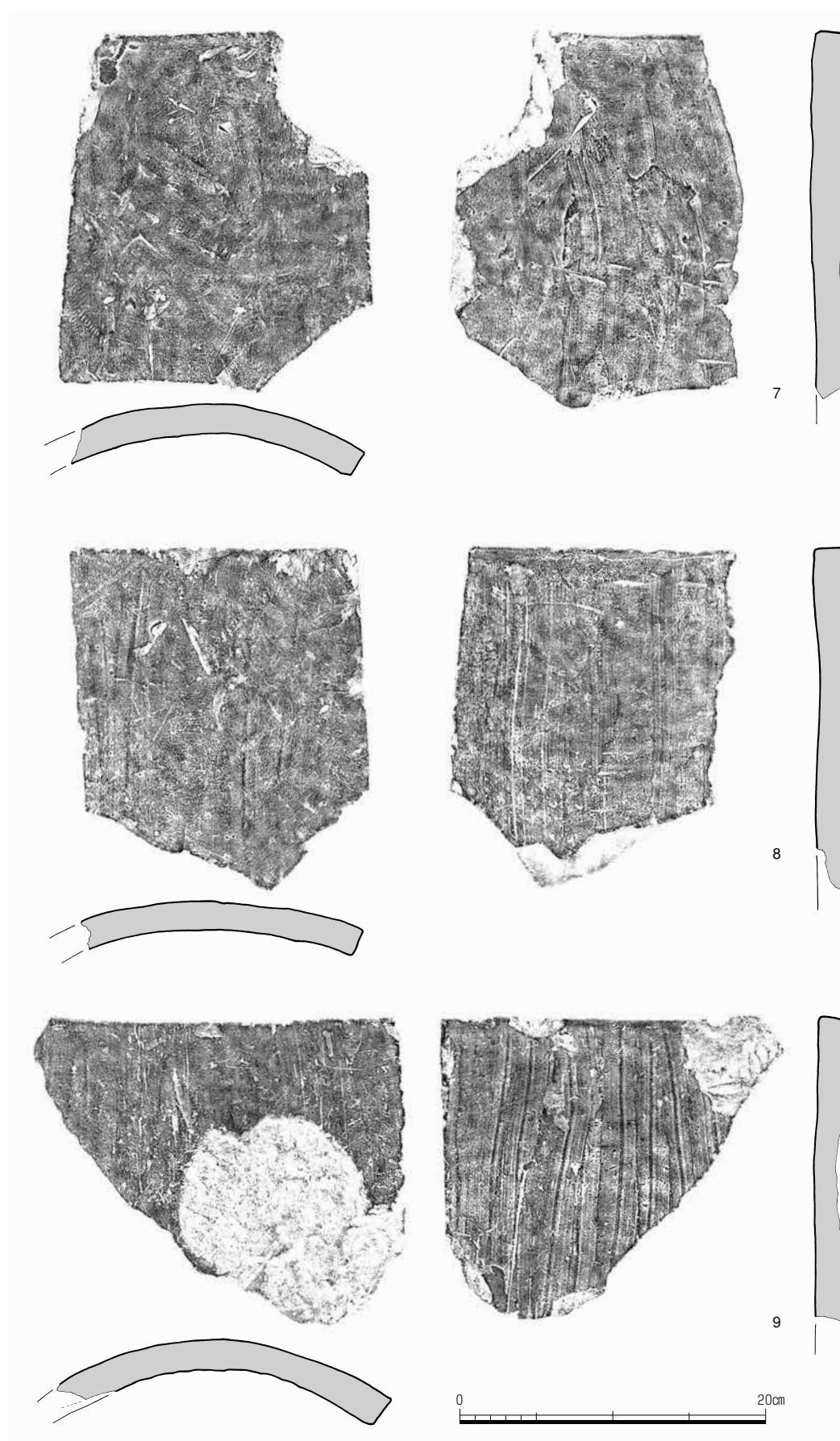
Fig. 76 平瓦1類拓影(2) 1:4
