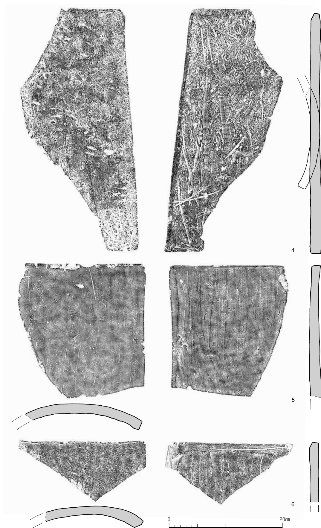
Fig. 75 平瓦 1 類拓影 (1) 1:4
