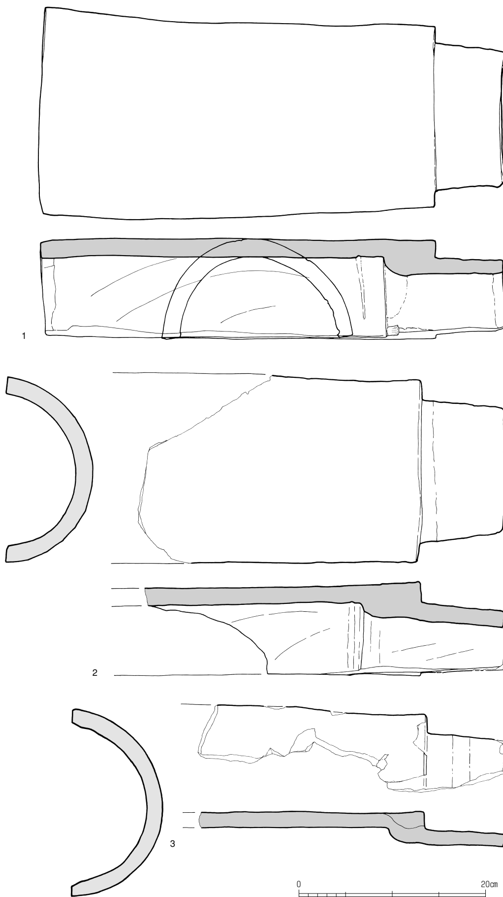
Fig. 67 丸瓦実測図 (1) 1:4
