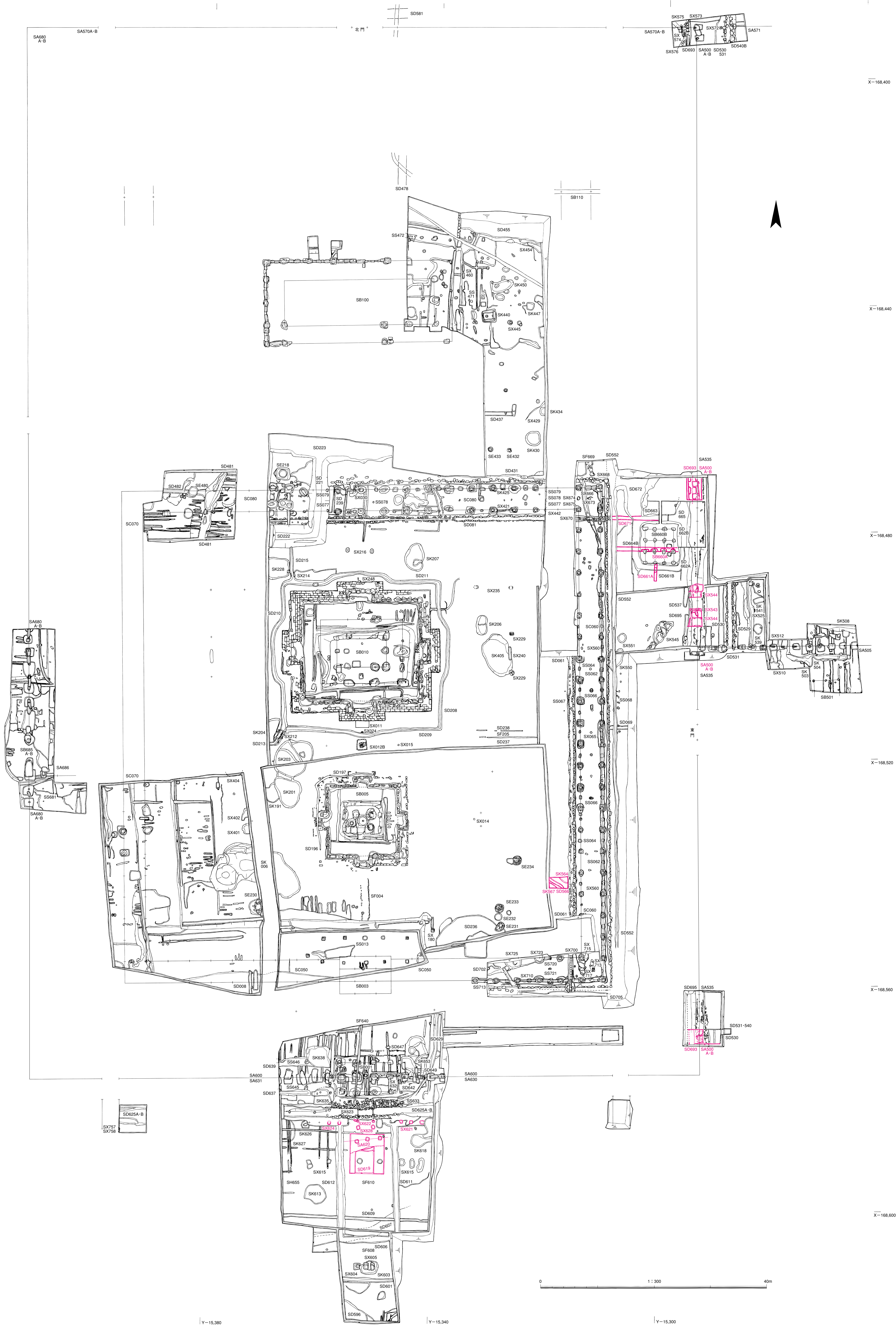
付図 1 山田寺遺構全図
