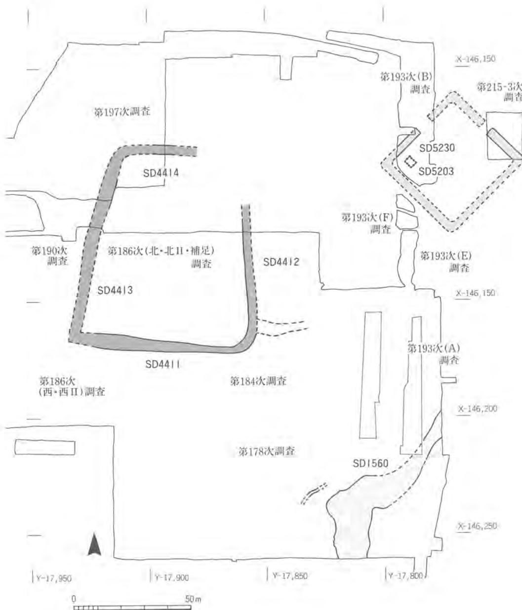
Fig. 40 居館復原図 1 : 1600
