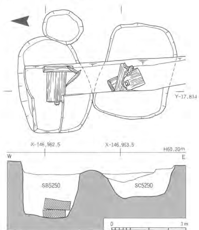
Fig. 45 SB5250とSC5290の柱穴と礎板 1 : 30
