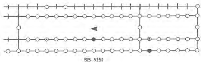
Fig. 45 SB5250とSC5290の柱穴と礎板 1 : 30
