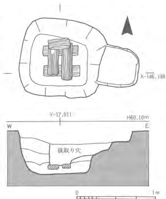
Fig. 32 SB4490の柱穴と礎板 1:30
