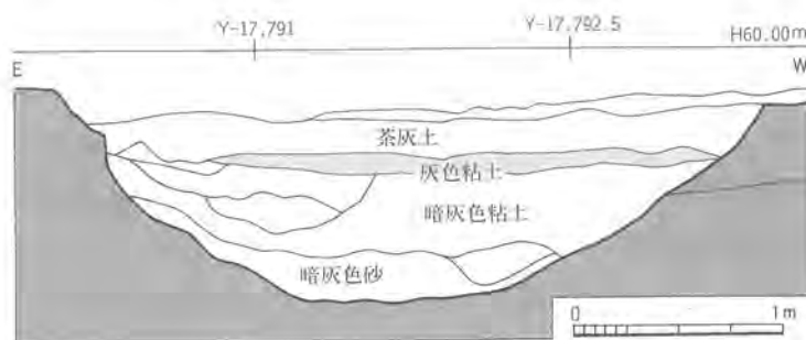
Fig. 23 SD4699土層図 1:40
