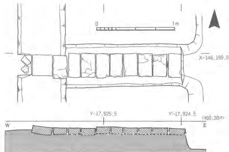
Fig.37 暗渠SX4555B実測図 1:30
