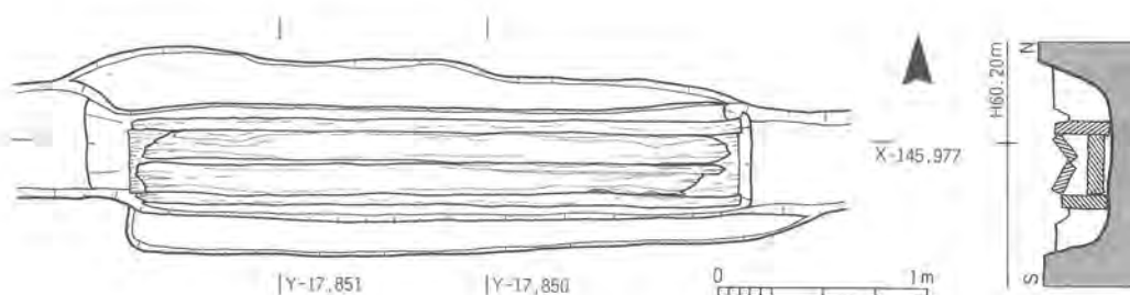
Fig. 42 暗渠SX5336実測図 1 : 40
