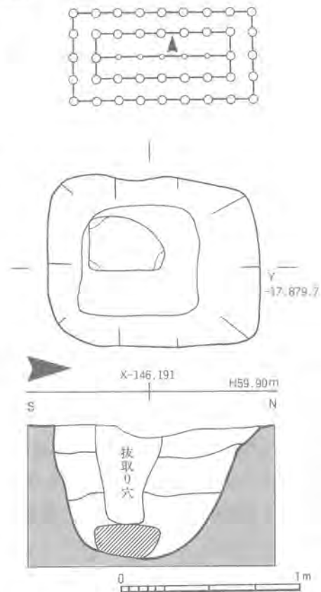
Fig.35 SB4300の柱穴と礎板 1:30
