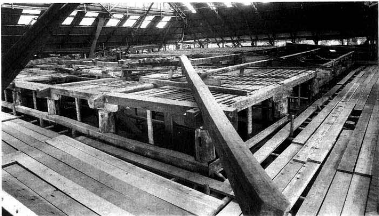
図V-8 解体修理中の重要文化財大直禰子神社本殿
