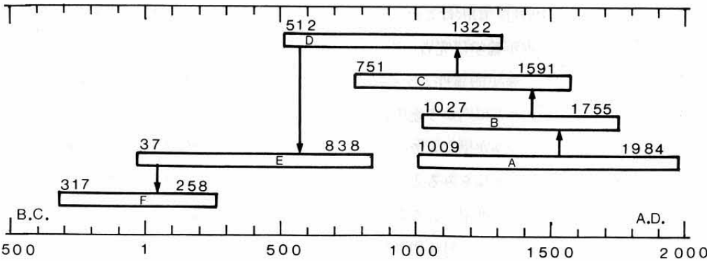
図V-2 6組のヒノキの暦年標準パターン
