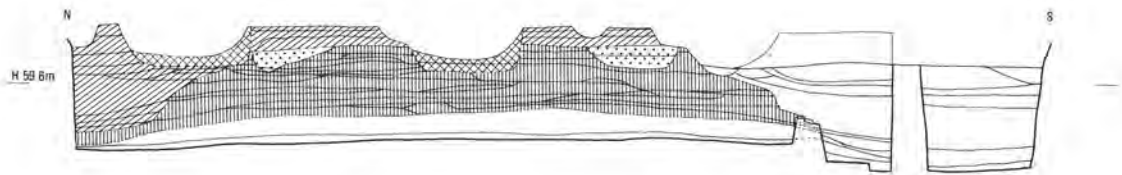
A. 南面回廊南北断面
