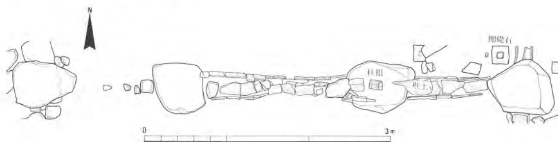
西僧房大房（7房）南入側詳細
