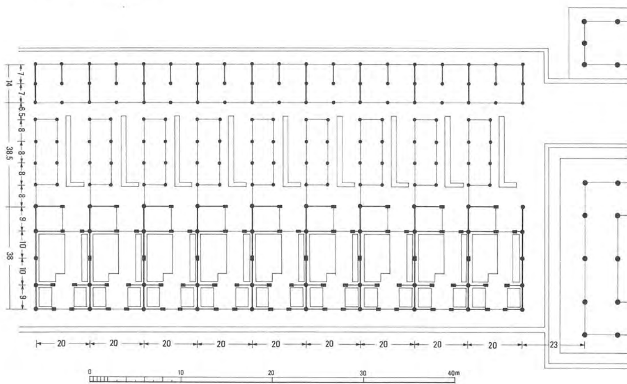
西僧房平面模式图
