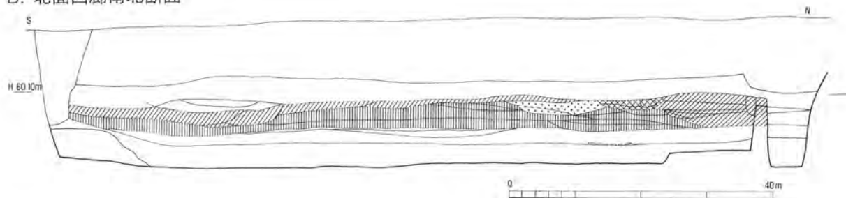
B. 北面回廊南北断面
