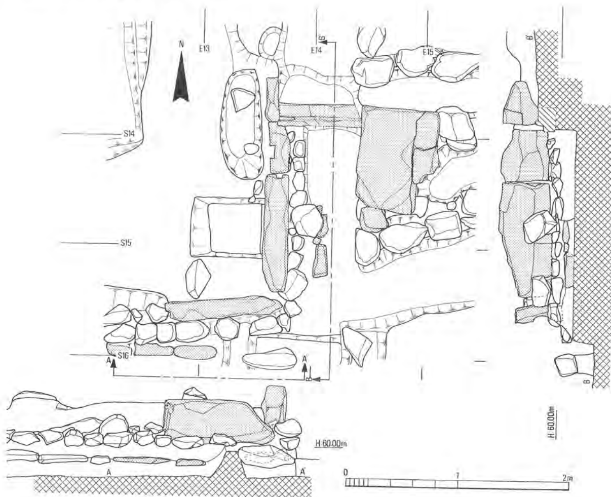
中門東南入隅部基壇外装平面・立面図
