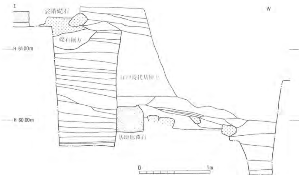
基壇断面土層図(基壇東端)
