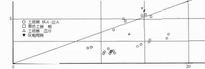
12 虎鷄山1号窯灰釉陶器法量分布表
