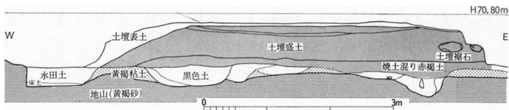
Fig. 11 お旅所土壇東西断面図
