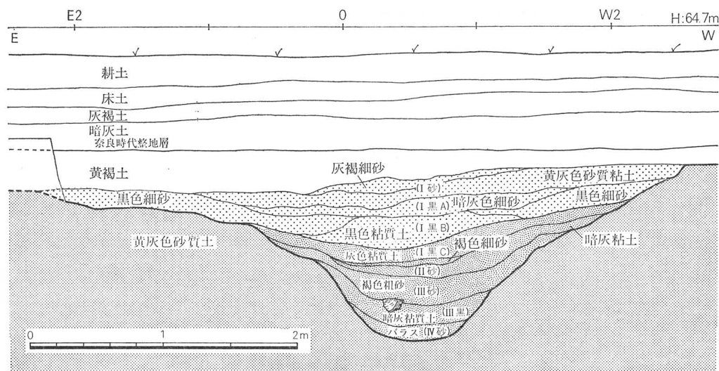
Fig. 6 SD6030 北区土層図
