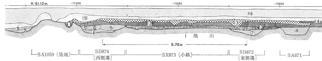
fig. 7 SX873断面図
