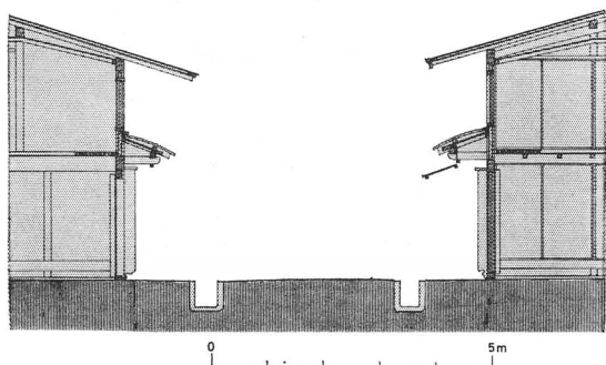
3-5 恵比須台組 道路と町家の関係 (上 復原、下 現状)
