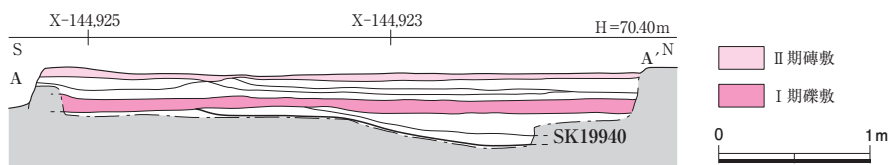
図126 東区A-A' ライン土層図 1 : 50
