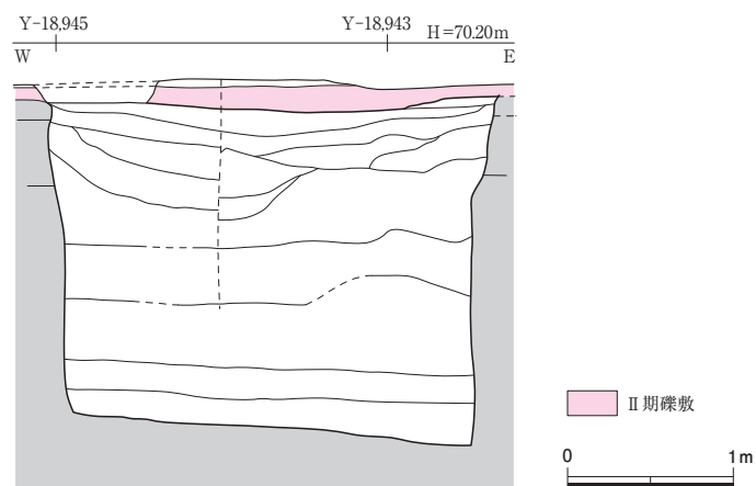
图128 土坑SK19945断面图 1 : 50
