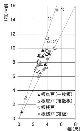
図4 古代建築の扉の大きさと形式
