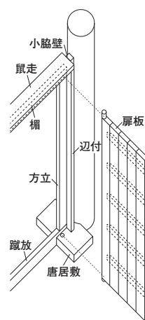
図5 扉構え模式図(朱雀門参考)
