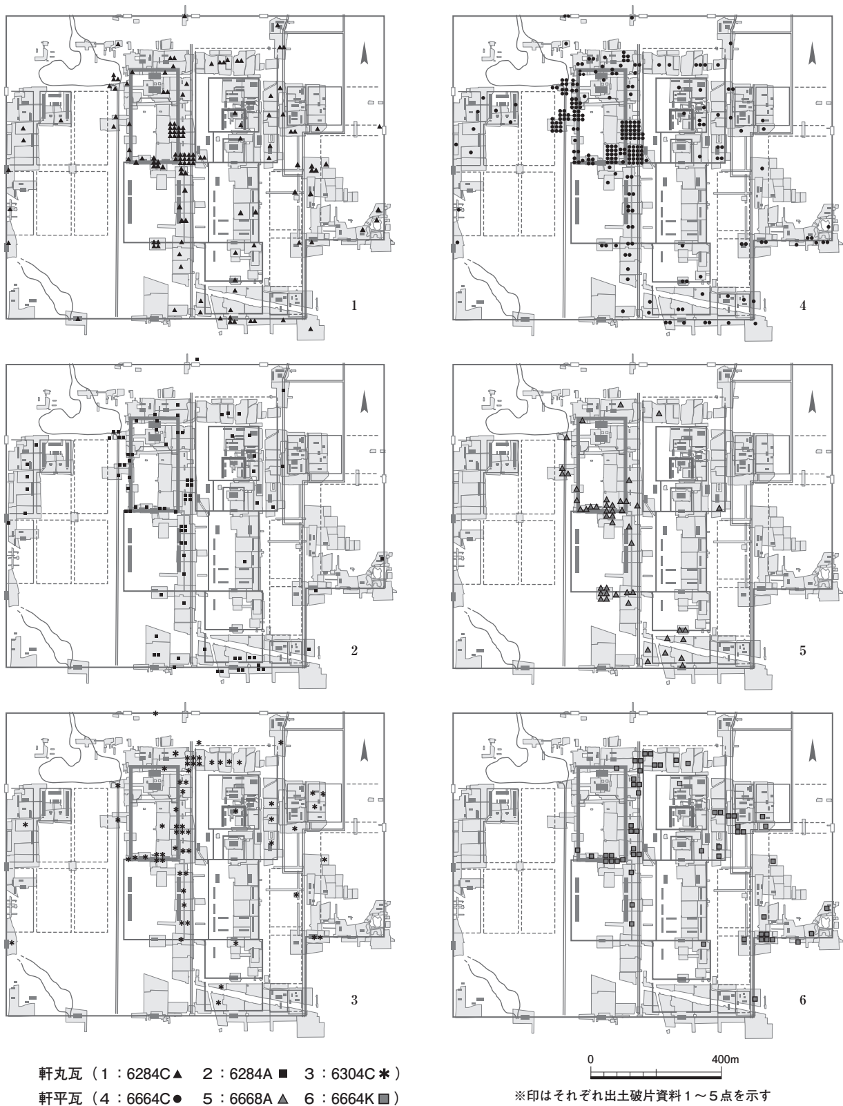
図3 第一次大極殿院造営にかかわる軒瓦の平城宮内出土分布
