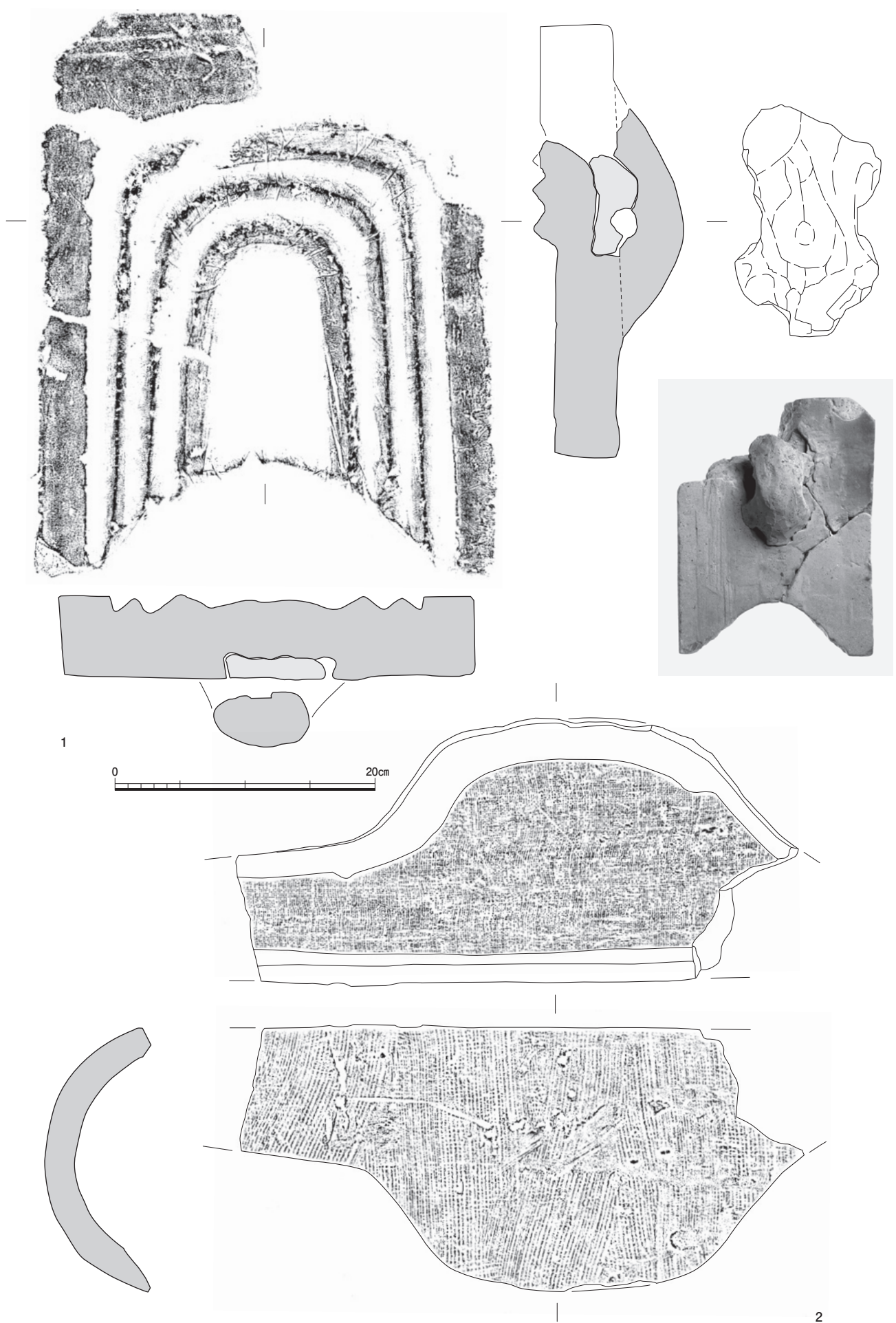
図Ⅱ-59 SD170出土の鬼瓦とSK11121出土の面戸瓦 1 : 4
