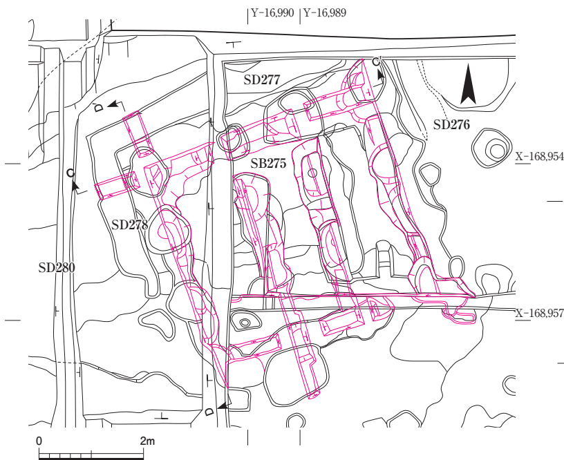
図 II-41 建物SB275遺構平面図・断面図 1 : 100
