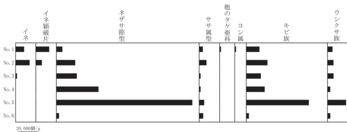
図 II-51 谷埋立土における植物珪酸体分布図
