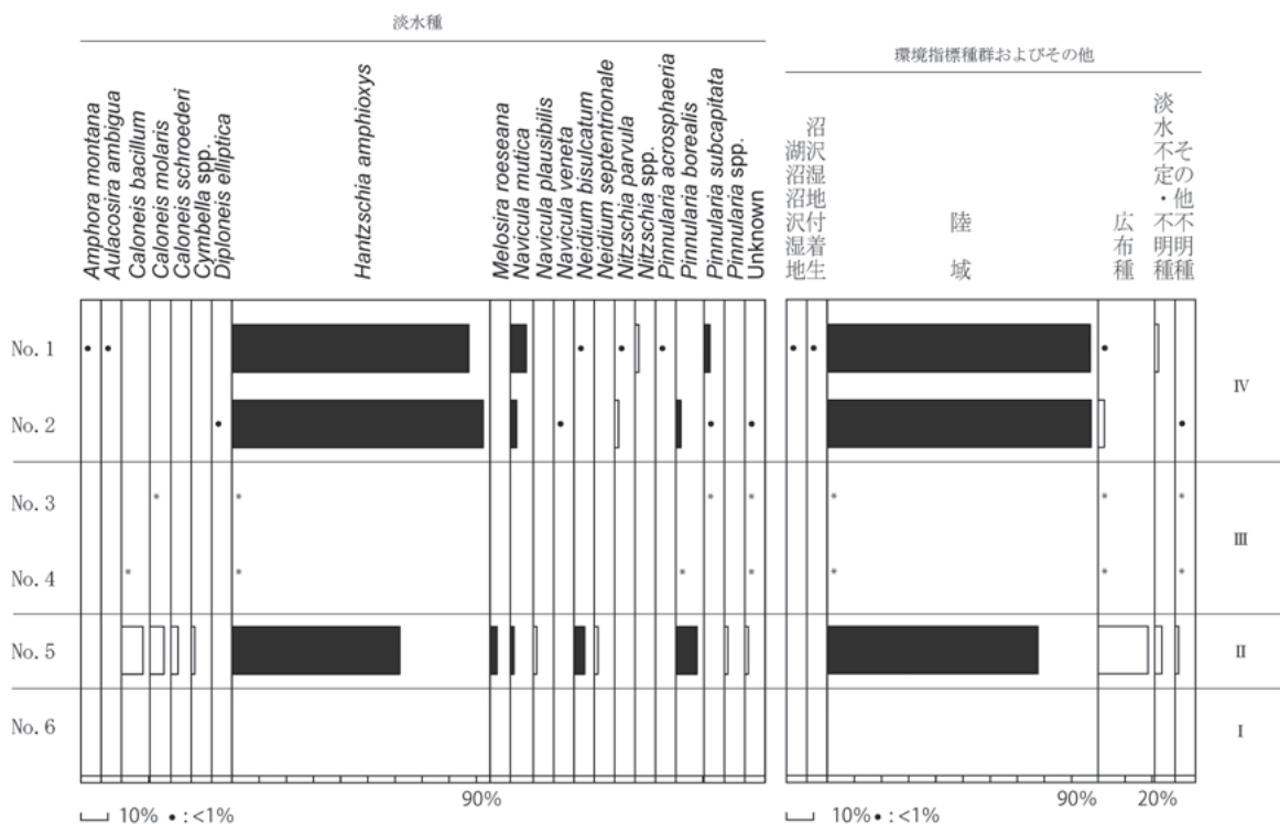
図 II-52 谷埋立土における珪藻化石分布図
