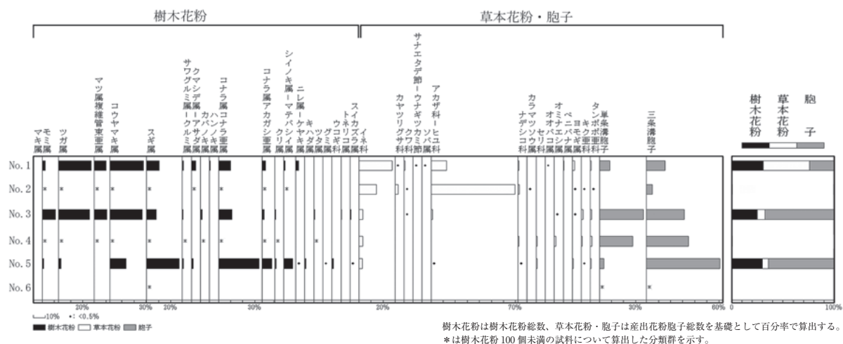
図 II-50 谷埋立土における花粉分布図
