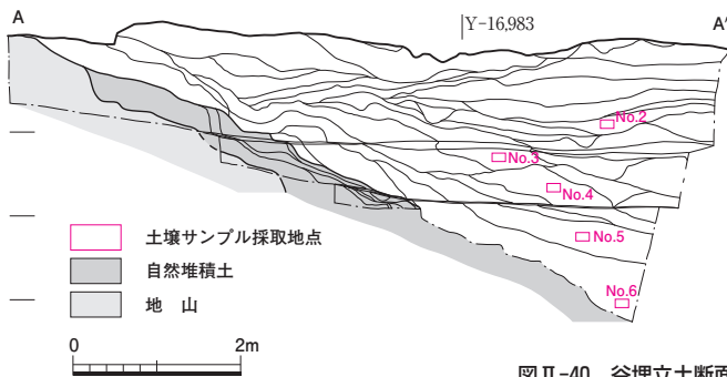
図 II-40 谷埋立土断面図 1 : 100
