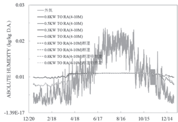
図 I-53 石室内空氣の絶対湿度の年変化
