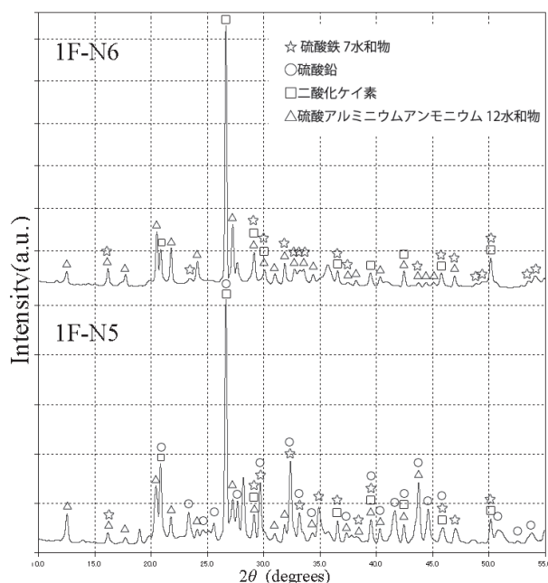
図 I-45 1F-N5と1F-N6のXRDチャート
