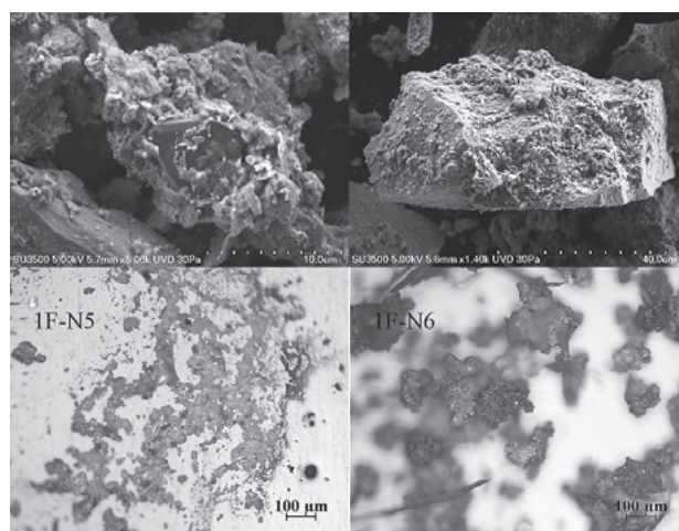
図 I-44 1F-N5と1F-N6の色料粒子
