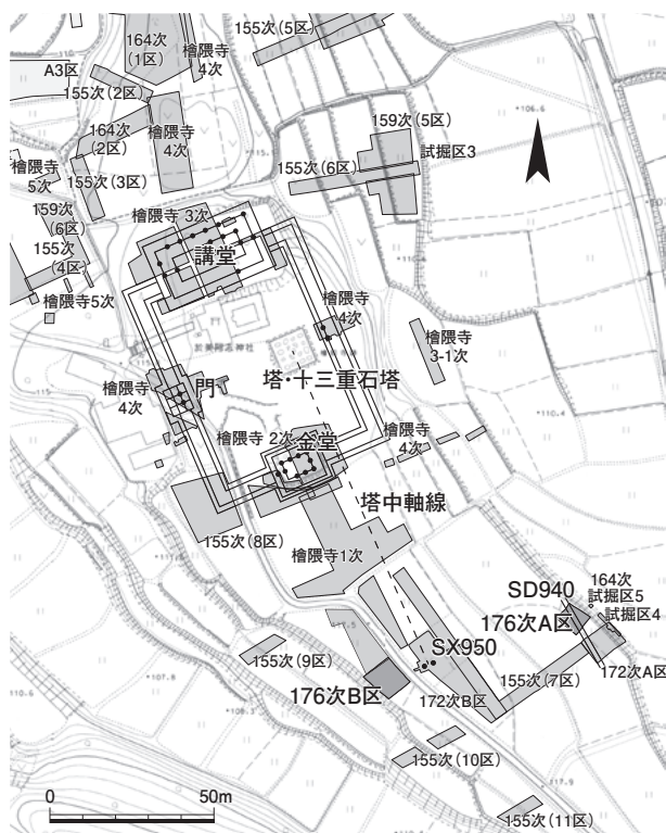
図166 第176次調査区位置図と主な遺構 1：2500
