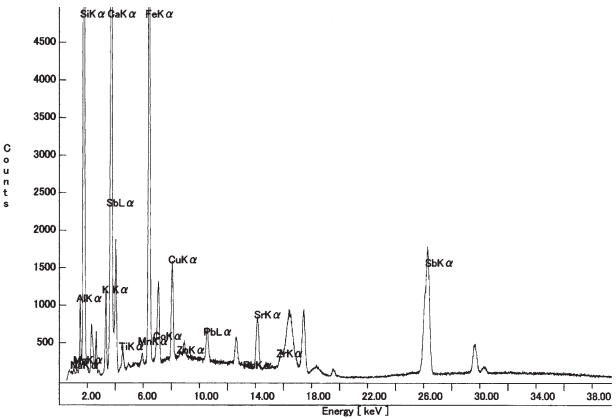
図89 蛍光X線スペクトル(分析No.2)
