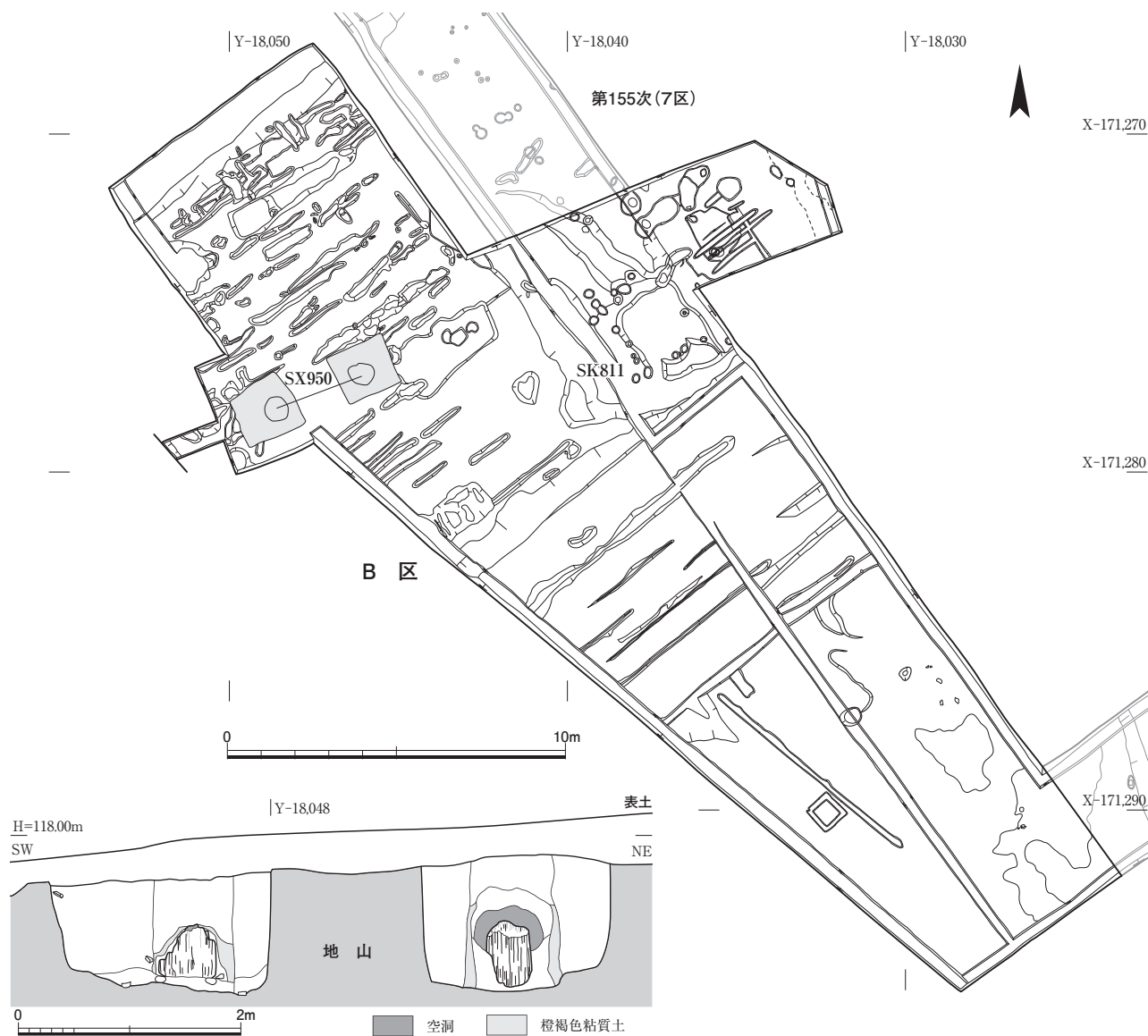
図181 SX950断面図 1:60
