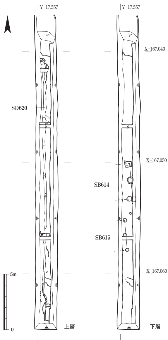
図113 北5区遺構図 1:200
