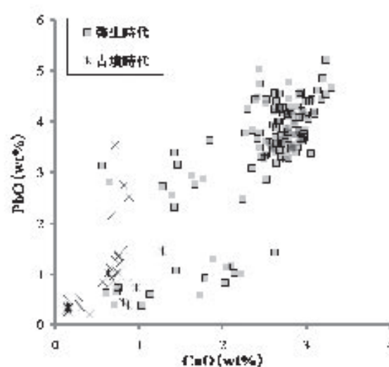
図47 黄緑色ガラス小玉の \text{CuO} - \text{PbO} 量
