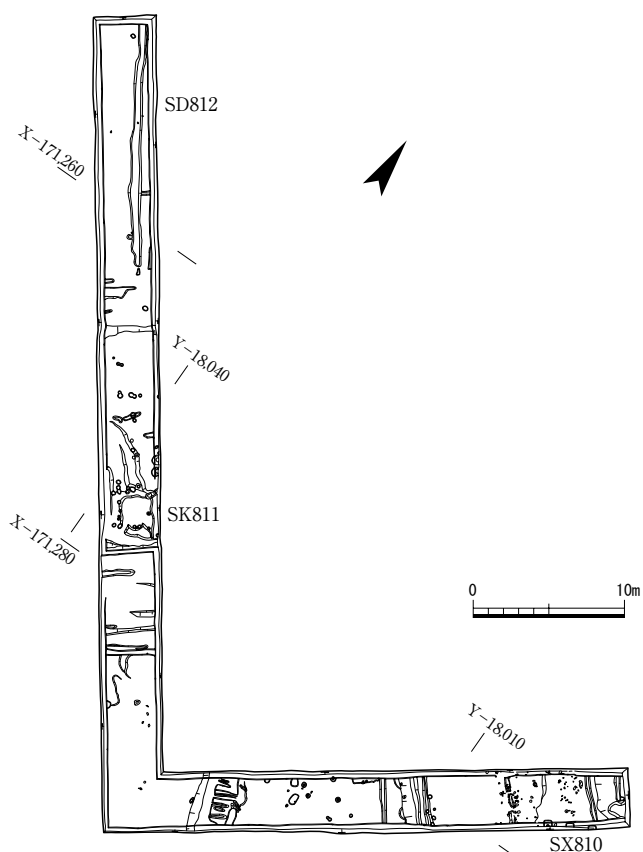
図119 第8区遺構図 1 : 300
