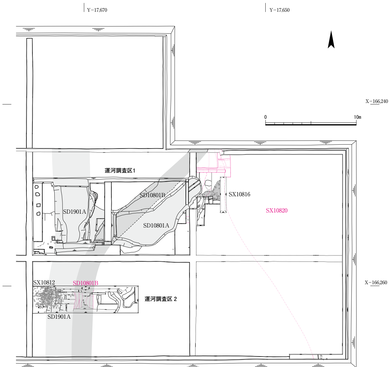
図55 第153次調査宮造営期遺構図 1 : 250
