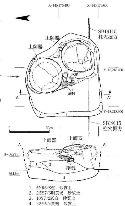
図43 SK19121平面図・断面図 1:10
