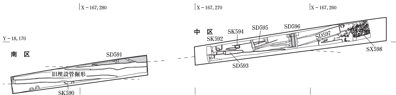
図91 第149-7次調査遺構図 1:200
