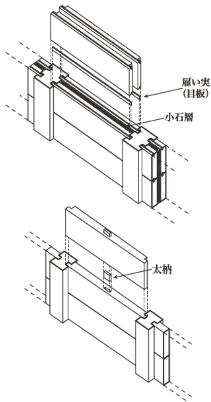
図85 壁模式図 (上:堀内家文庫蔵、下:有賀家土蔵)
