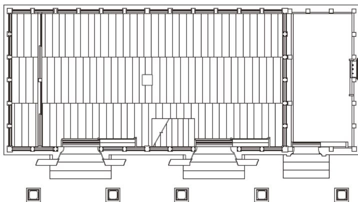
図83 堀内家文庫蔵 1:150 (左:1階平面図、右:梁行断面図妻面筋)
