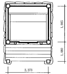
図76 命主社平面図 1 : 100
