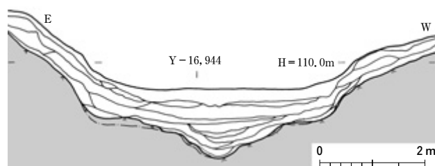
図91 SD4195南壁土層断面図 1:1000
