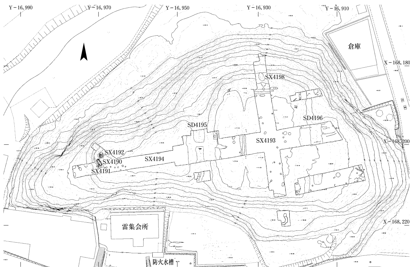
図90 第139次地形測量図と遺構平面図 1:600
