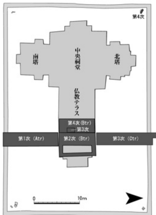
図1 西トップ寺院の調査位置図 1:500
