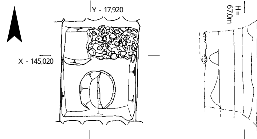
図189 SD8702実測図 1 : 40
