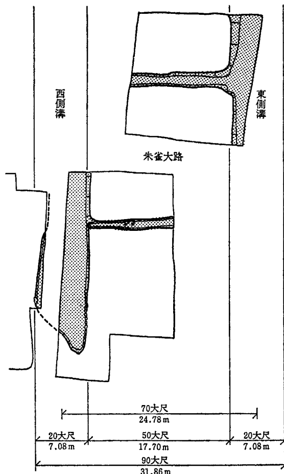
図87 藤原朱雀大路設定復元図 1:500 (注6 井上論文より)
