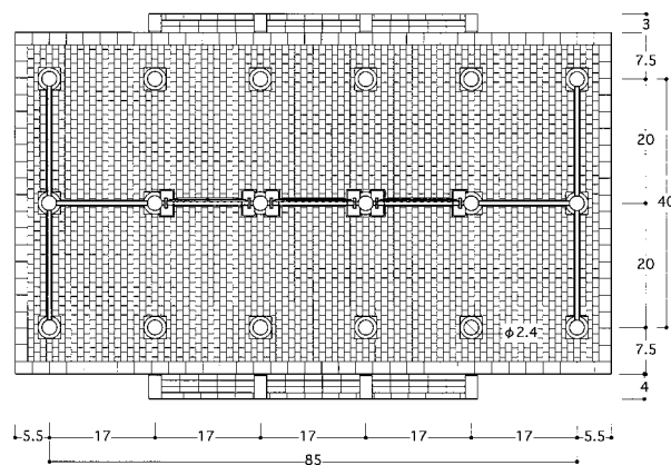
図44 南門梁間2間単層門案 平成14年度案 1:400
