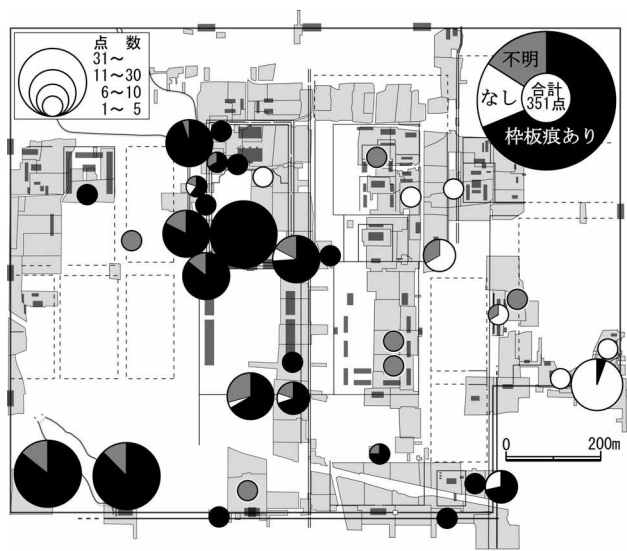
図36 平城宮の熨斗瓦出土状況
