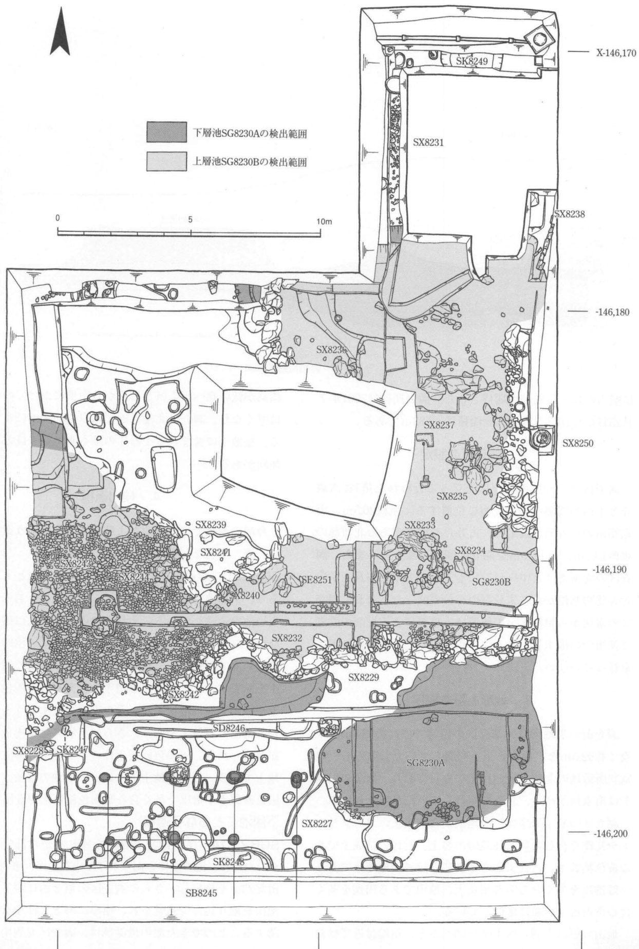
図112 第330次調査遺構平面図 1:150
