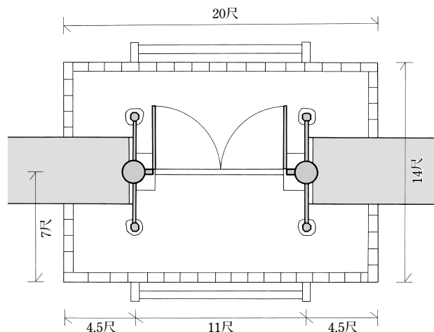
図156 SX850四脚門案復原図 1:100 (浅川滋男による)
