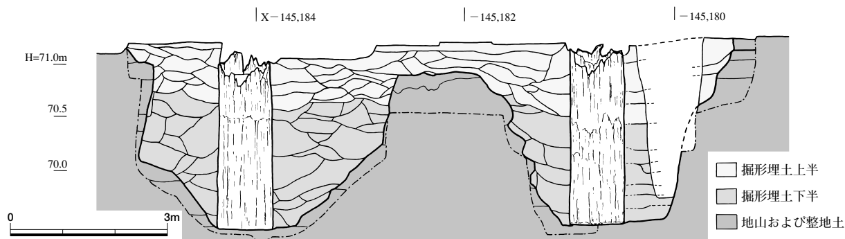
図153 SX850断面図 (Y=-19,574.5) 1:50
