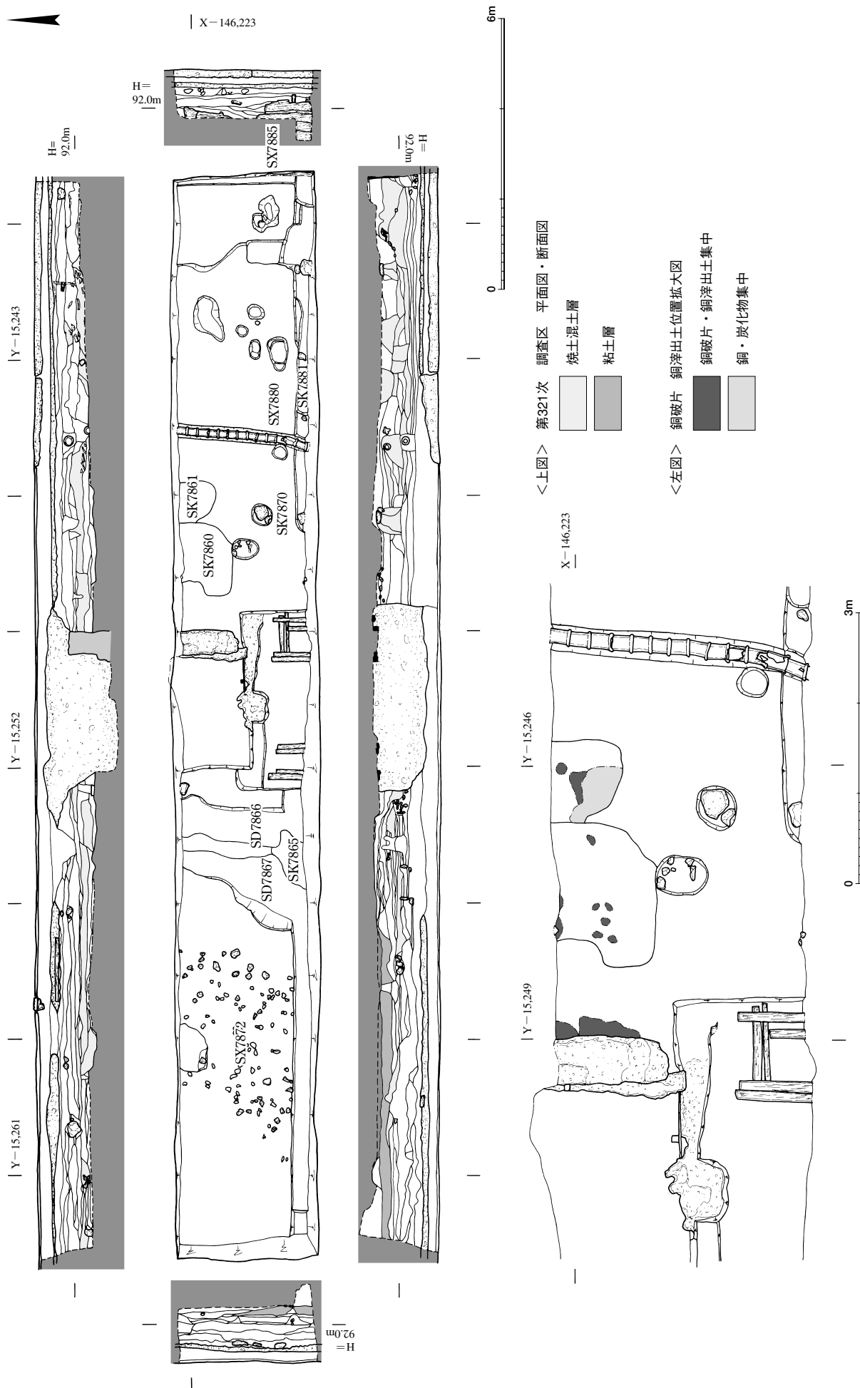
図133 第321次調査遺構平面図・断面図(左) 1:120、銅破片・銅滓出土位置拡大図(右) 1:60
