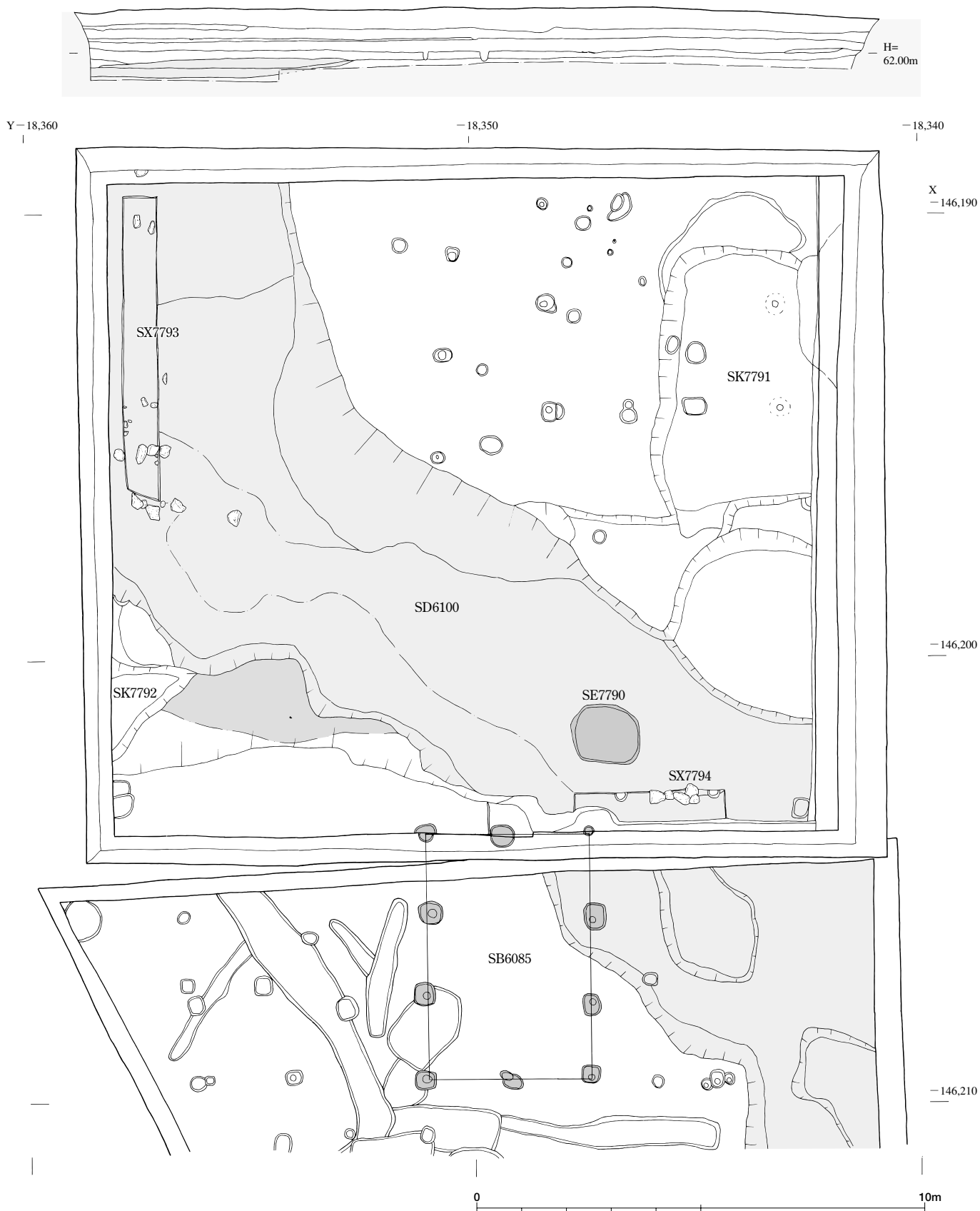
図124 第314-7次遺構平面図・北壁断面図 1:120
