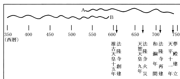
図49 法隆寺夢殿桁材 (A) および (B) の年輪成長曲線 (西岡氏原図)
