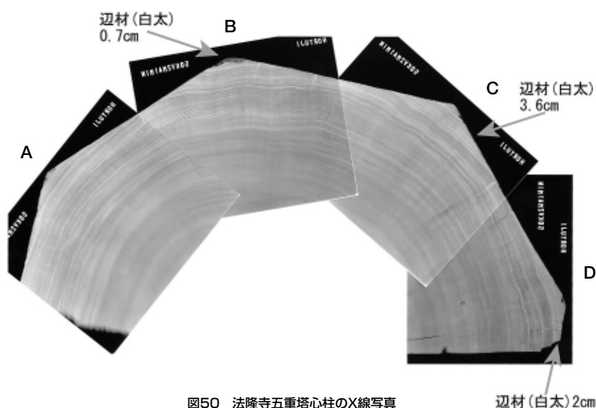
図50 法隆寺五重塔心柱のX線写真
