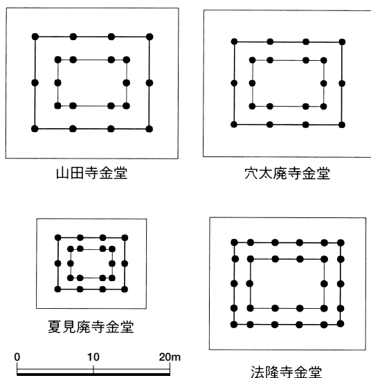
図20 山田寺金堂他平面図
