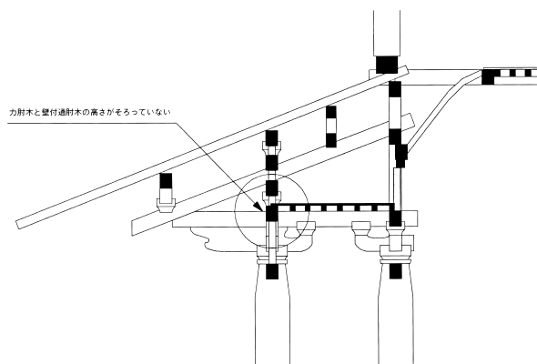
図21 法隆寺金堂組物断面図
