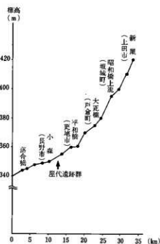
図2 千曲川の断面図〔『更埴市史』一部改変〕
