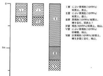
基本層序模式図
