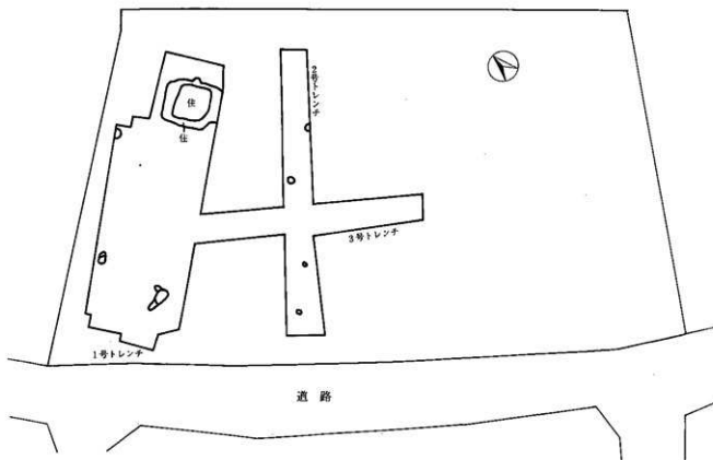
試掘トレンチ設定図 (1 : 300)
