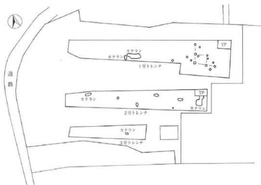
試掘トレンチ設定図 (1:500)
