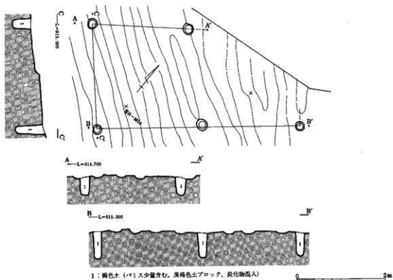
第383図 6号住居址・1号掘立柱建物址
