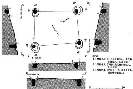
第384図 2・3号掘立柱建物址
